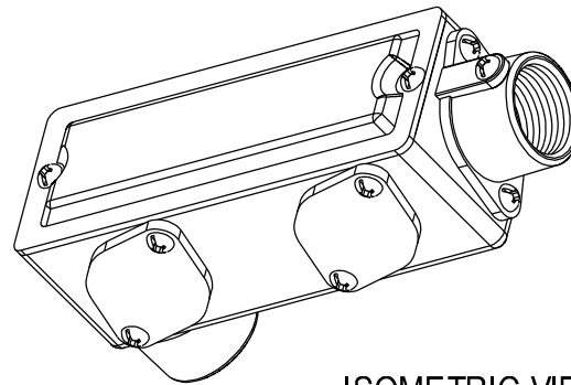
ISOMETRIC VIEW (SCALE:NONE)
