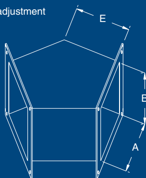
45° ELBOW
