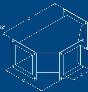
TEE
