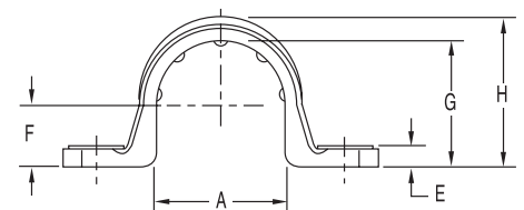
Conduit Clamps
