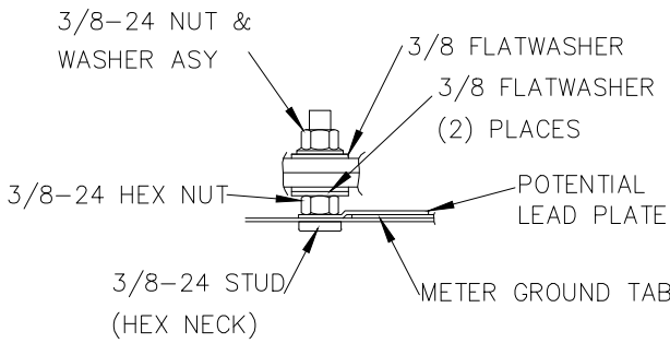
NEUTRAL STUD DETAIL
