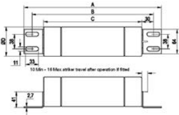
F Tags
