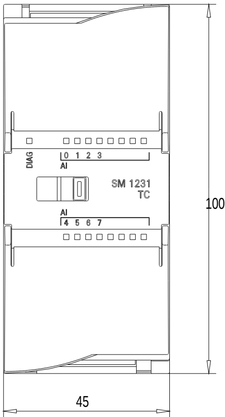
Vorne / Front
