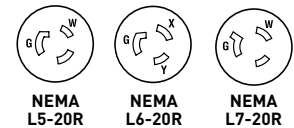
20A Connector
