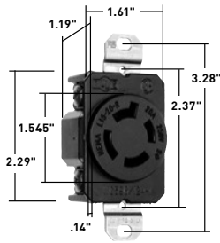
20A Receptacle
