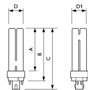
PL-C ALTO 13W/835/4P
