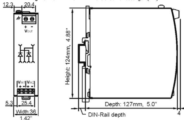
Fig. 9 / Bild 9 YR40.482: Dimensions / Abmessungen (mm)
