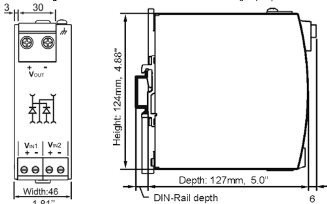
Fig. 10 / Bild 10 YR80.241: Dimensions / Abmessungen (mm)
