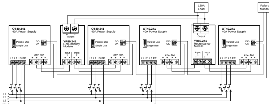
Typical N+1 redundant system with four 40A power supplies for load current up to 120A Typisches N+1 redundantes System mit vier 40A Stromversorgungen für Ströme bis zu 120A
