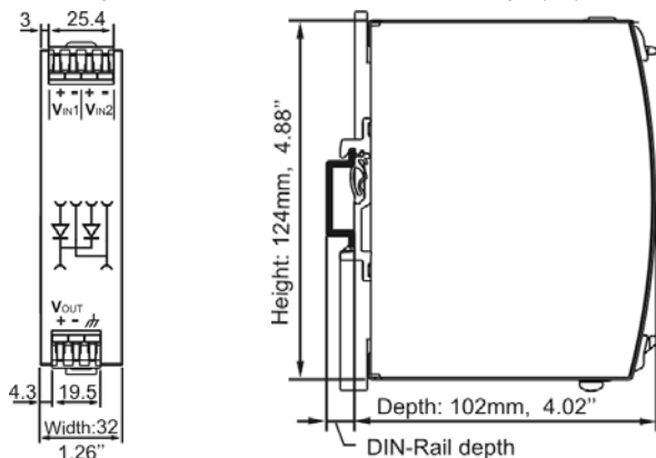
Fig. 6 / Bild 6 YR40.241: Dimensions / Abmessungen (mm)
