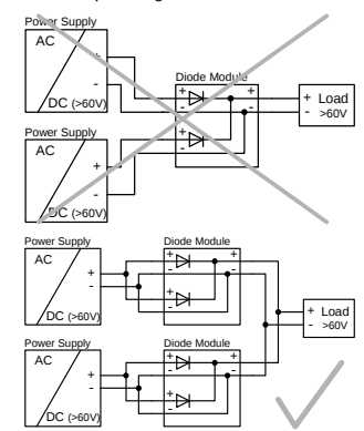
Fig. 3 / Bild 3 YR2.DIODE: Utilizing voltages between 60 and 150Vdc/ Betrieb mit Spannungen zwischen 60 und 150Vdc
