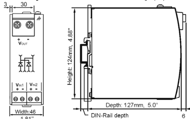
Fig. 11 / Bild 11 YR80.242: Dimensions / Abmessungen (mm)
