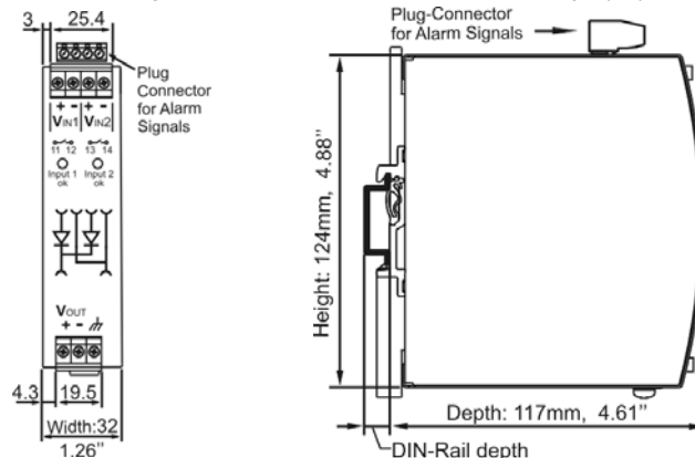
Fig. 7 / Bild 7 YR40.242: Dimensions / Abmessungen (mm)
