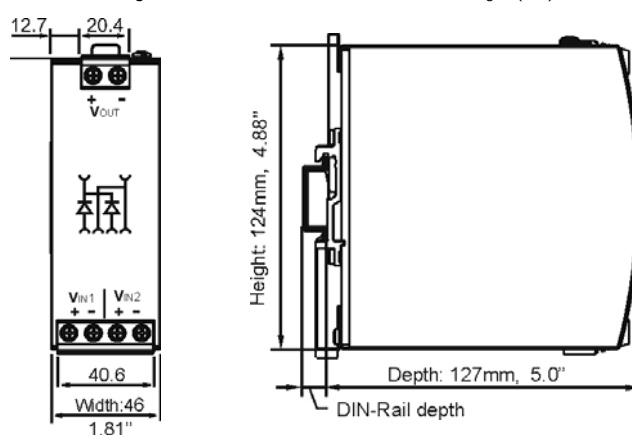
Fig. 11 / Bild 11 YR80.242: Dimensions / Abmessungen (mm)
