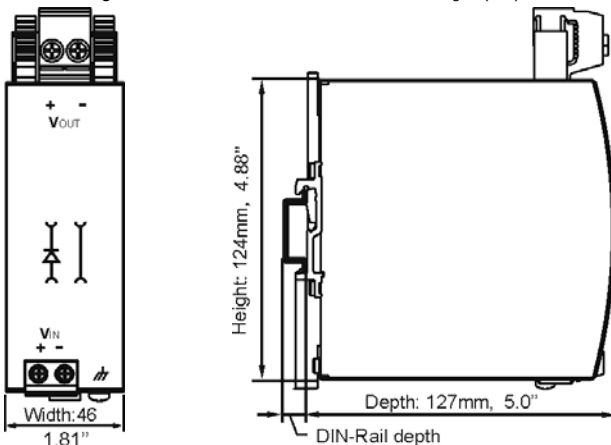
Fig. 10 / Bild 10 YR80.241: Dimensions / Abmessungen (mm)
