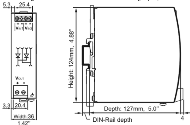
Fig. 8 / Bild 8 YR40.245: Dimensions / Abmessungen (mm)
