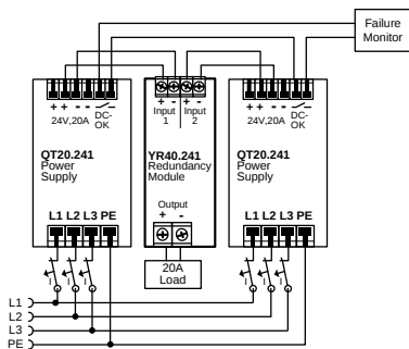
Typical 1+1 redundant system for load currents up to 20A Typisches 1+1 redundantes System für Ströme bis zu 20A
