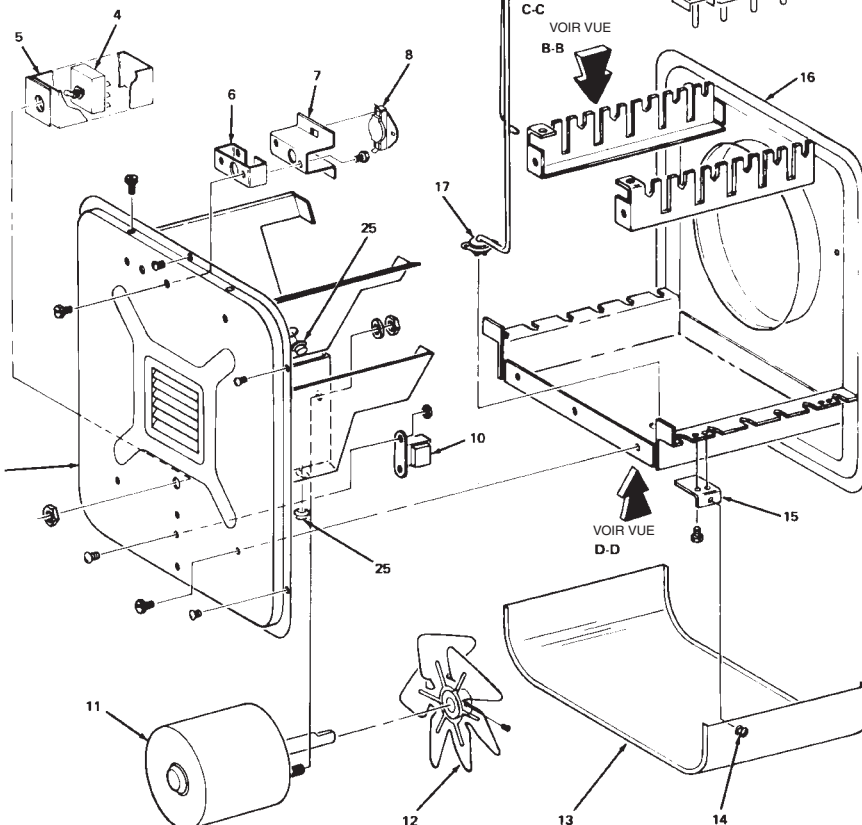
VUE C-C
