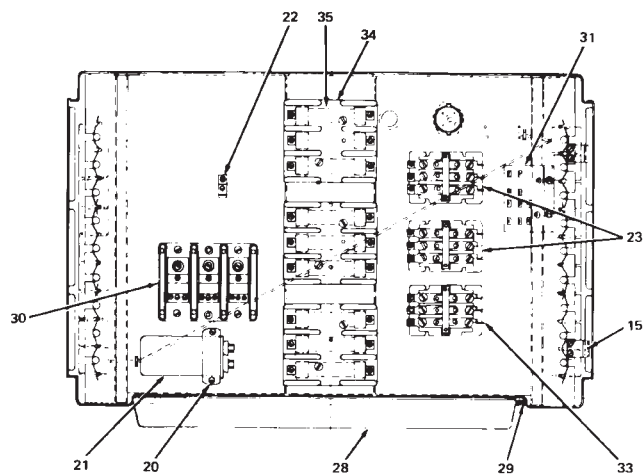
VISTA D-D (MUH -25 HASTA MUH 50 SOLAMENTE)
