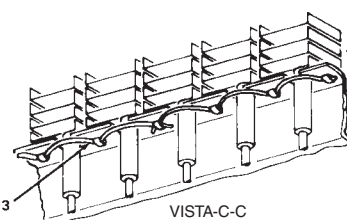
VISTA C-C
