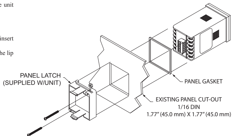
1/16 DIN Installation
