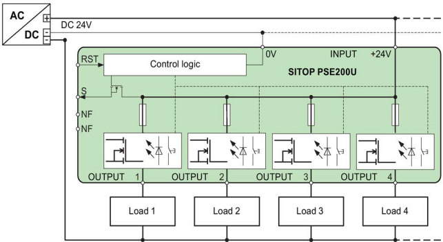
Bild 10: Blockdiagramm 6EP1961-2BA61 Figure 10: Block diagram 6EP1961-2BA61 Figura 10: Diagrama de bloques 6EP1961-2BA61 图 10: 框图 6EP1961-2BA61 Figure 10: Schéma fonctionnel 6EP1961-2BA61 Figura 10: Diagramma a blocchi 6EP1961-2BA61 Рисунок 10: Блок-диаграмма 6EP1961-2BA61
