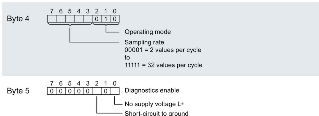
Figure A-16 Module parameter block
