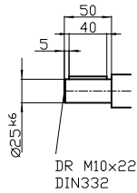
DIN 6885-1
