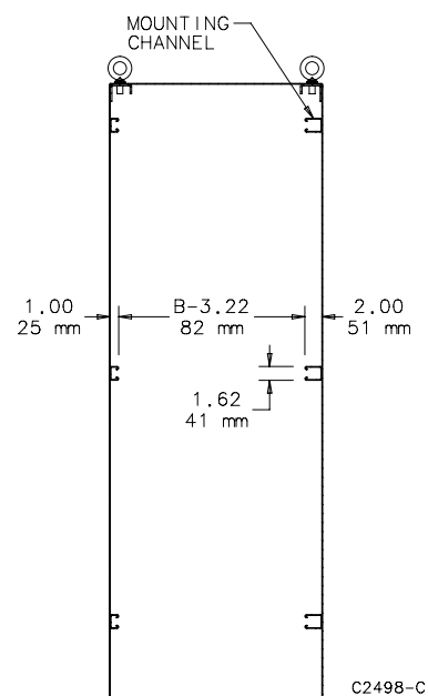
SECTION A-A
